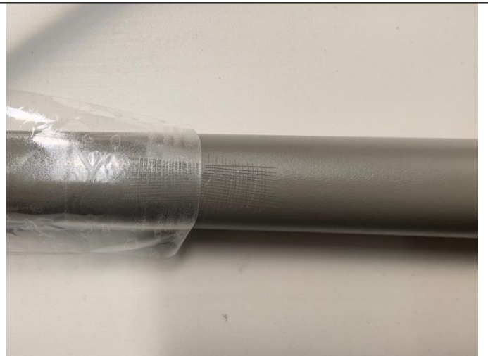
百格测试
