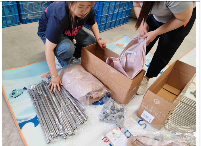
摔箱测试
