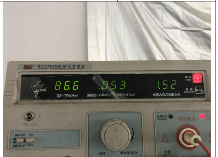
Hi-pot test
