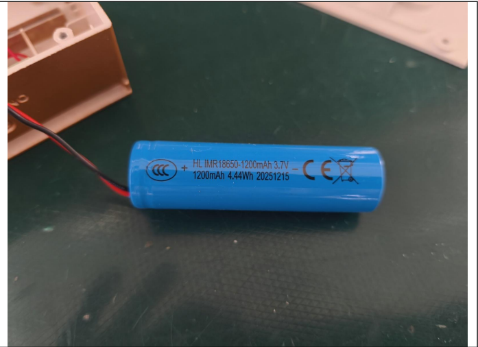
电池细节
