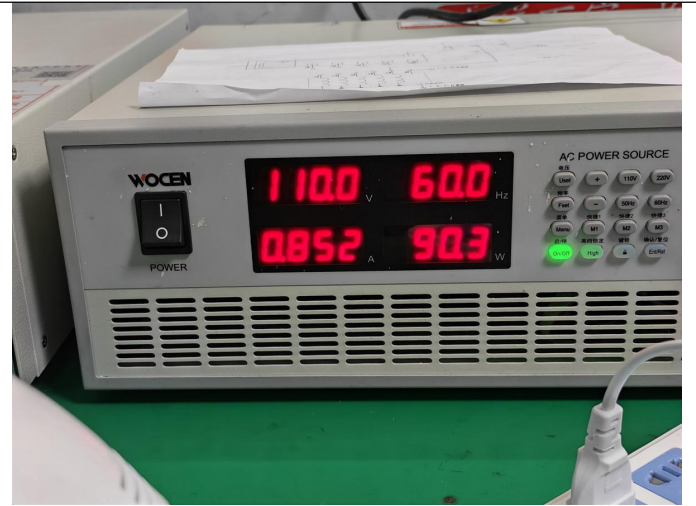
2 档功率 90.3W
