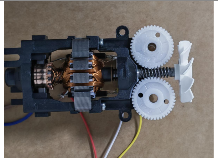
拆机检查
