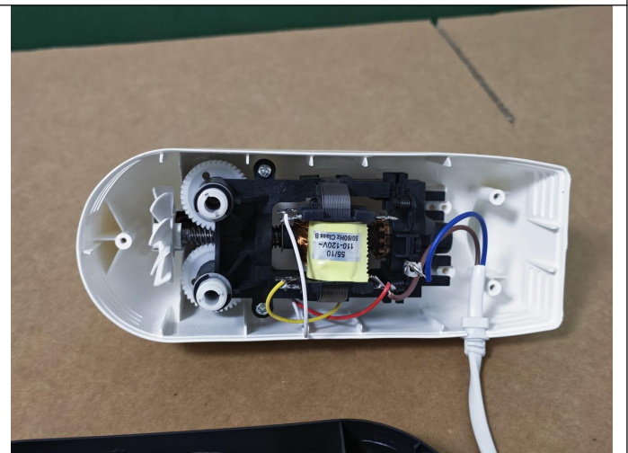
拆机检查
