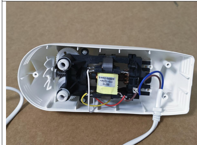
拆机检查
