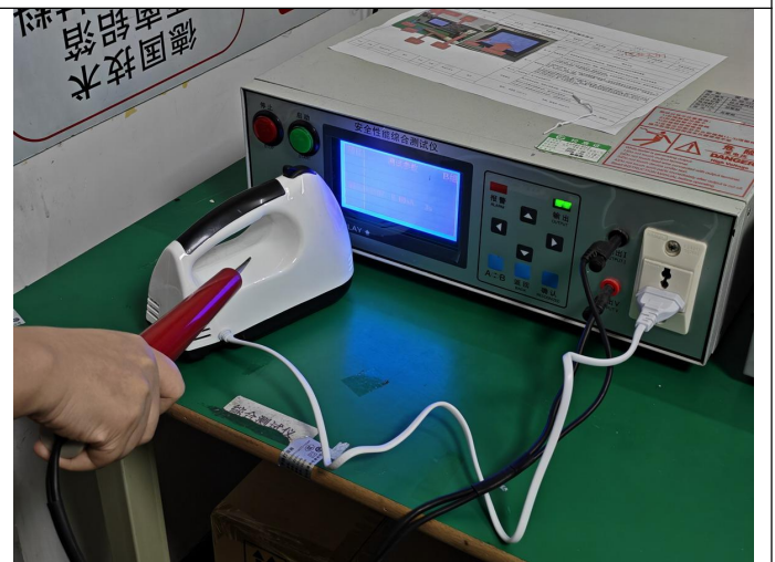
高压测试
