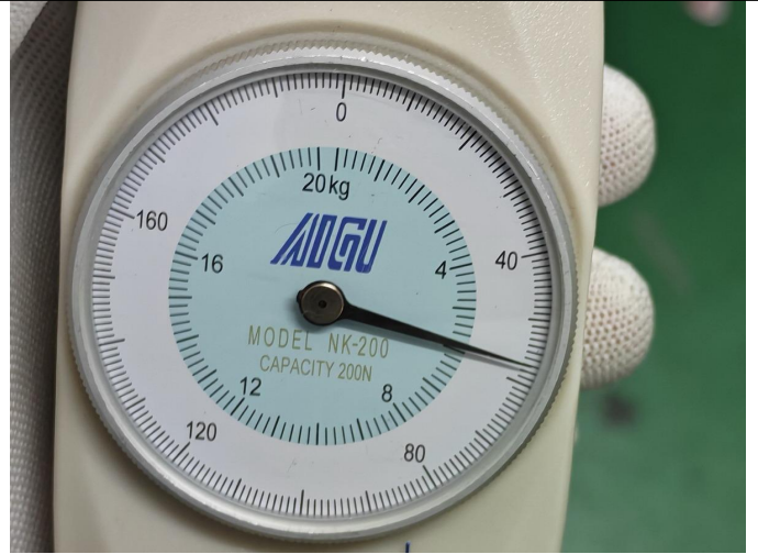
拉力测试 58.5N
