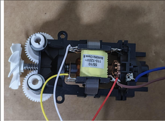
拆机检查
