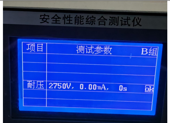
高压测试 电压 2750V 3 秒
