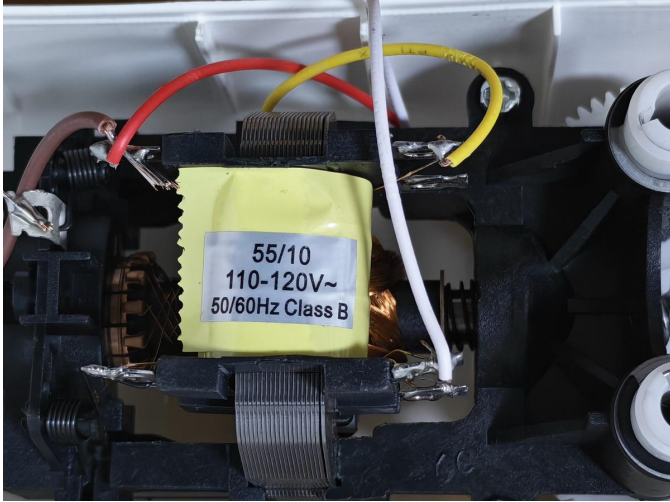
拆机检查
