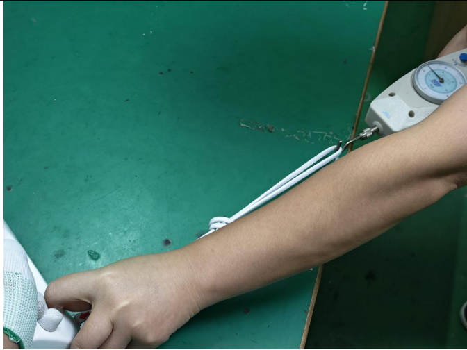
拉力测试
