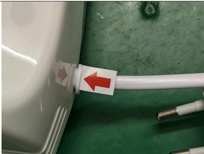
拉力测试
